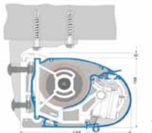
Top Fix
